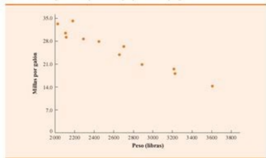
FIGURA 16.8 Diagrama de dispersión del ejemplo de millas por galón
